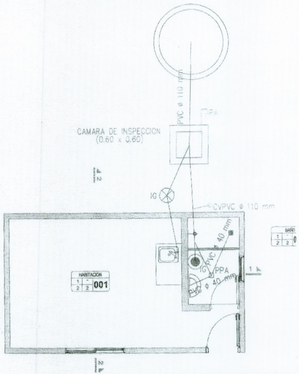
PLANTA SANITARIA escala 1:50
