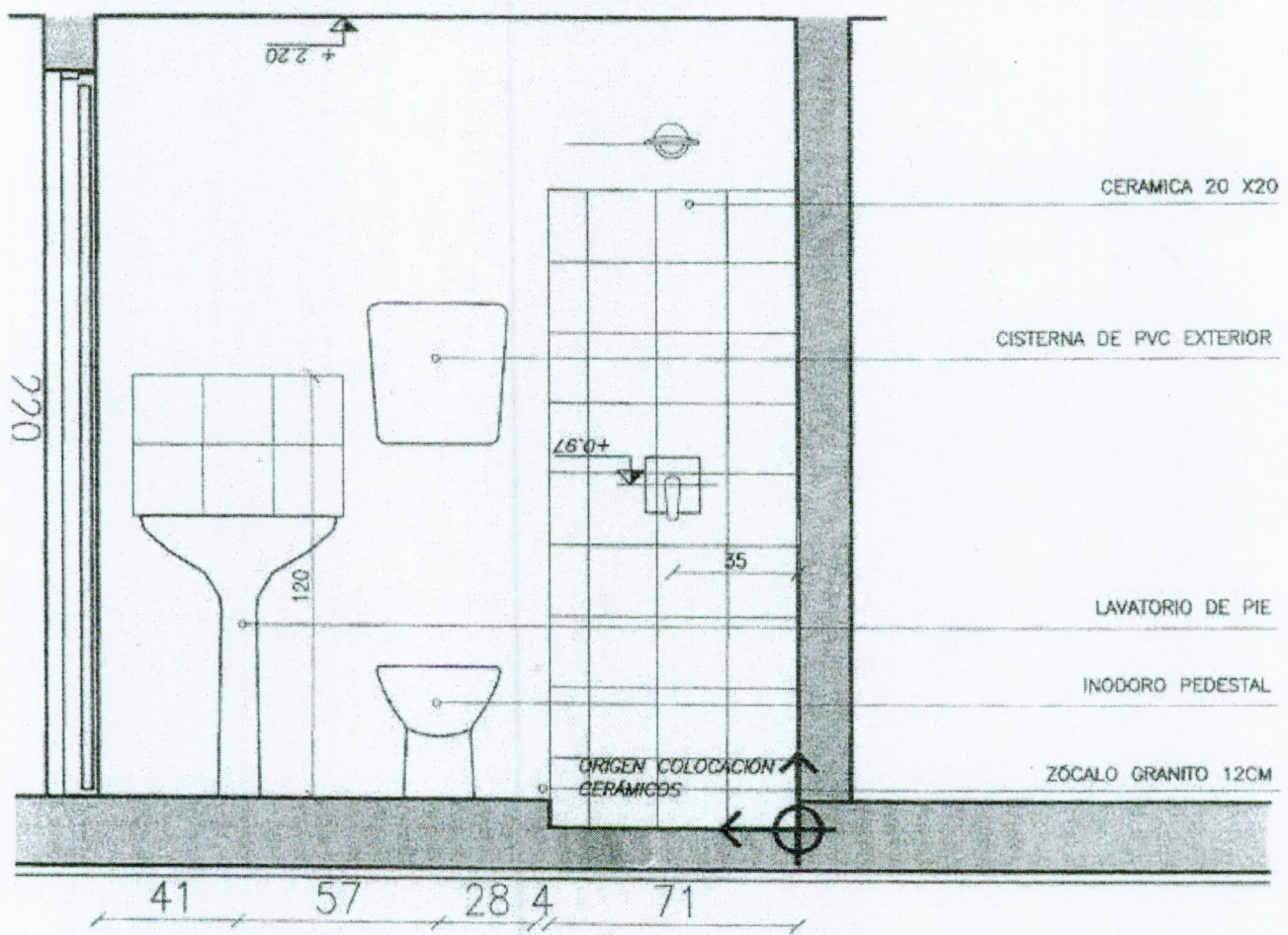
VISTA 4-4 ESC.1/20
