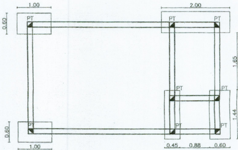
PLANTA FUNDACION escala 1:50
